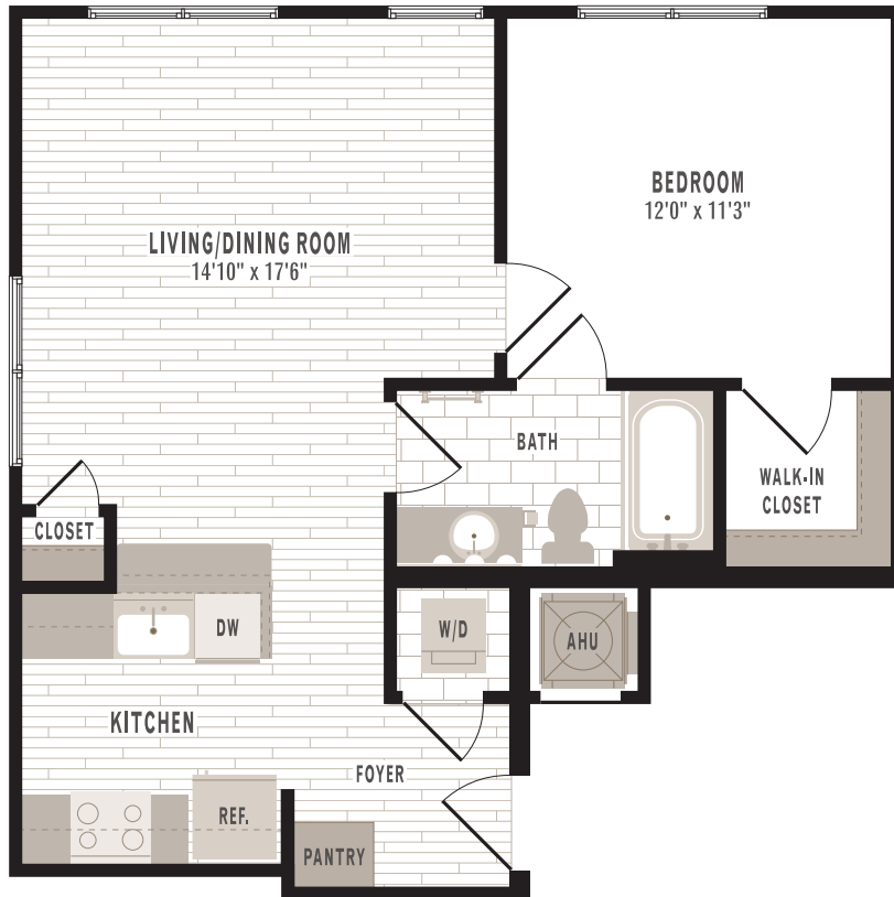
UNIT A5
